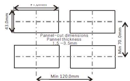
판넬 가공
